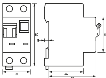
Maßzeichnung FI-/LS-Kombinationen DRCBO 3 B32/0,03/1N-A
