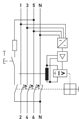
Schaltungsbeispiel FI-/LS-Kombinationen DRCBO 4 C16/0,10/3N-PV
