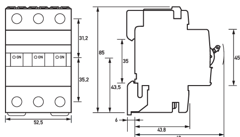
Maßzeichnung Leitungsschutzschalter DLS 6hsl B6-3
