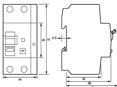
Maßzeichnung FI-/LS-Kombinationen DRCBO 4 B20/0,03/1N-B+
