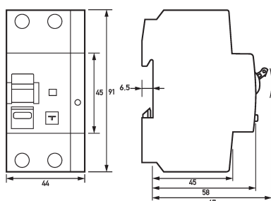
Maßzeichnung FI-/LS-Kombinationen DRCBO 4 B20/0,30/1N-B+
