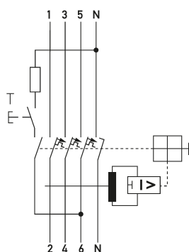
Schaltungsbeispiel FI-/LS-Kombinationen DRCBO 4 B40/0,30/3N-A
