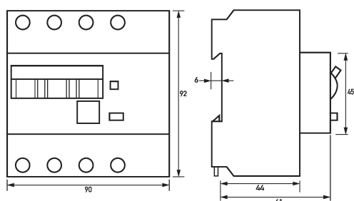
Maßzeichnung FI-/LS-Kombinationen DRCBO 4 B40/0,30/3N-A
