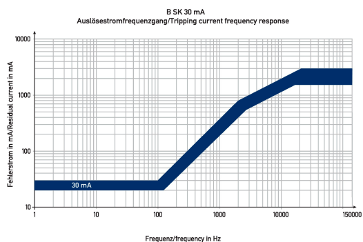
Diagramme FI-/LS-Kombinationen DRCBO 4 Bo6/0,03/1N-B SK
