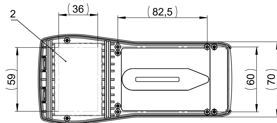
Oberschale / enclosure top
