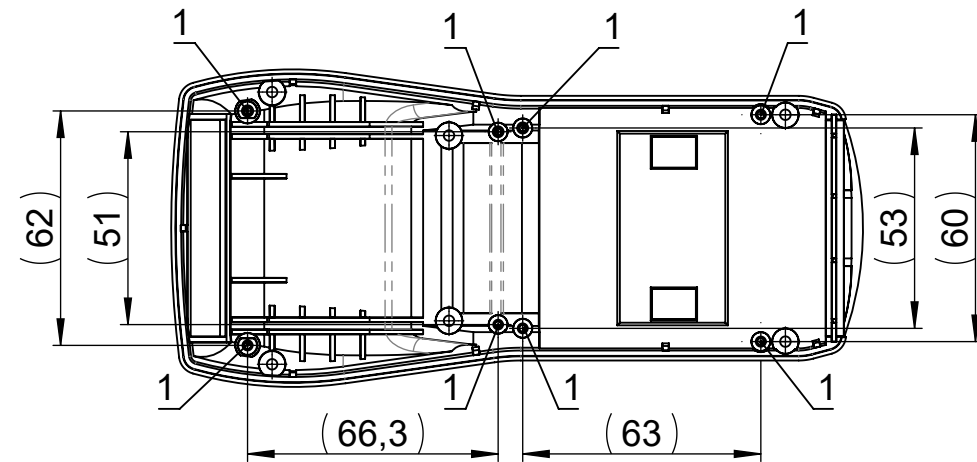
Unterschale / enclosure bottom
