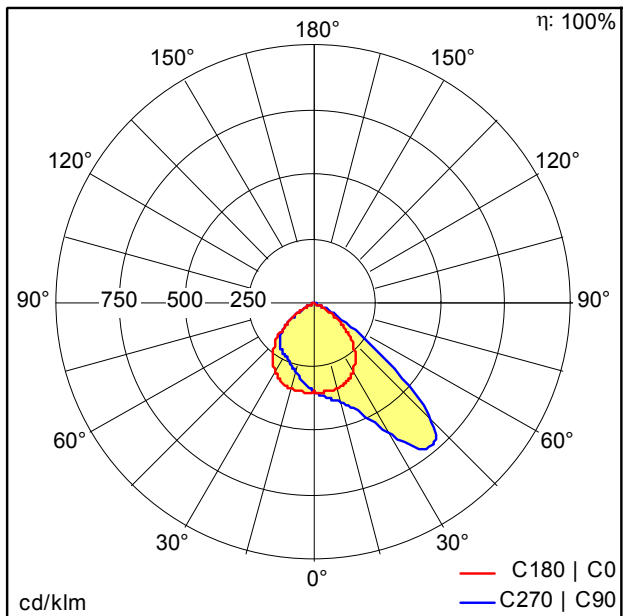
TE_LEO_LED_FL_IP66_100W_840_PC.ltd
