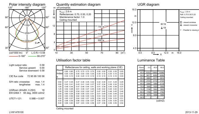
TCS640 2xTL5-49W HFP AC-MLO
