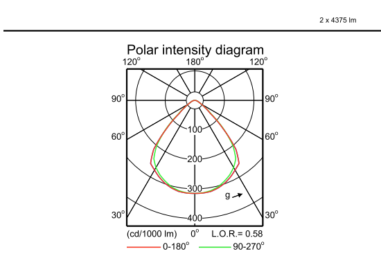
TCS640 2xTL5-49W HFP AC-MLO
