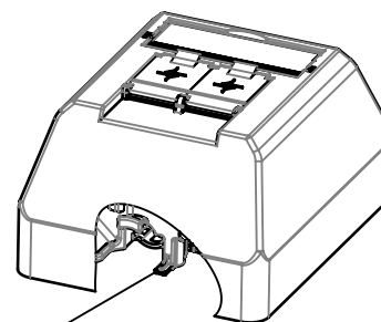
Flachstecker 2,8 mm DIN 46342-1 für Funktionserdung IEC 60364-5-54 Blade terminal 2,8 mm DIN 46342-1 for functional grounding acc. to IEC 60364-5-54
