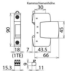
Maßbild DG S 75 FM
