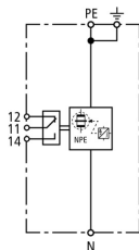
Prinzipschaltbild DGPM 440 FM
