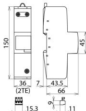
Maßbild DGPM 440 FM
