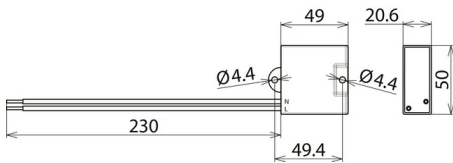
Maßbild DCOR L 1P 320
