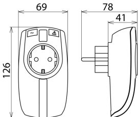
Maßbild DPRO 230
