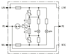
Prinzipialschaltbild DPRO 230
