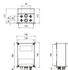
Maßbild DCU 2 YPV 1100 1M 1S MC4 FM
