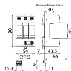
Maßbild DG M TNC 440 FM
