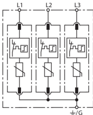
Prinzipialschaltbild DG MU 3PY 480 3W+G
