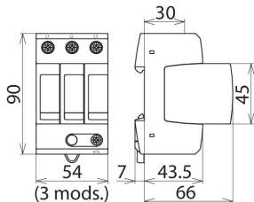
Maßbild DG MU 3PY 480 3W+G
