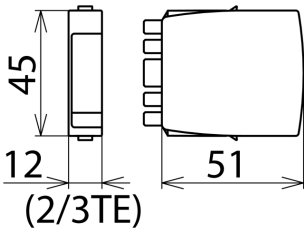
Maßbild BXT ML4 BE 5
