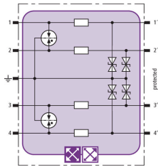
Prinzipschaltbild BXT ML4 BE 5
