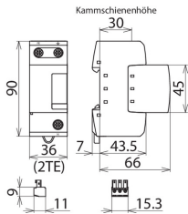
Maßbild DGP M 255 FM
