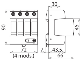
Maßbild DG MU 3PY 480 4W+G
