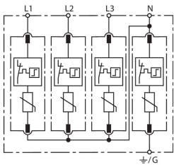
Prinzipialschaltbild DG MU 3PY 480 4W+G
