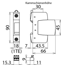
Maßbild DG S WE 600 FM
