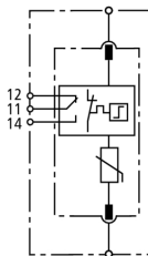
Prinzipialschaltbild DG S WE 600 FM
