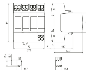
Maßbild DG MP TT 275 FM
