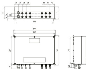
Maßbild DCU 2 YPV 1+2 1200 3M 1S MC4
