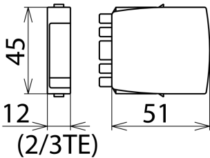
Maßbild BXT ML4 BE 24
