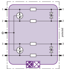
Prinzipialschaltbild BXT ML4 BD 12
