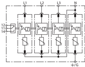
Prinzipschaltbild DG MU 3PY 208 4W+G R
