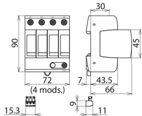
Maßbild DG MU 3PY 208 4W+G R
