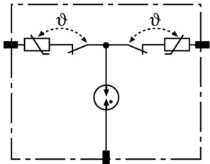
Prinzipschaltbild DR MOD 255
