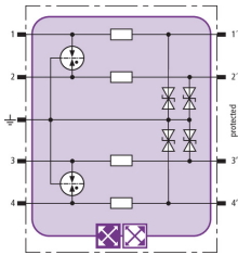
Prinzipschaltbild BXT ML4 BE 12
