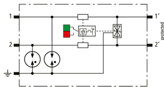
Prinzipschaltbild BCO ML2 BE HF 24
