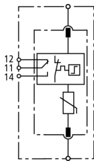
Prinzipschaltbild DG S 150 FM
