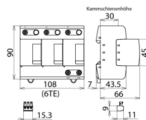
Maßbild DB MU 3PY 480 3W+G R
