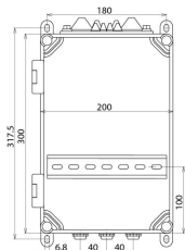
Maßbild IGA 10 V2 IP54
