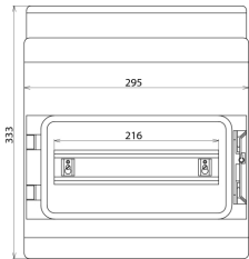
Maßbild IGA 12 IP54
