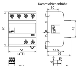
Maßbild DVA EMOB 3P 255 FM
