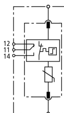
Prinzipialschaltbild DG S 440 FM
