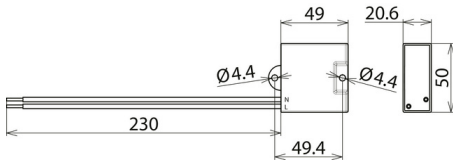
Maßbild DCOR L 1P 275
