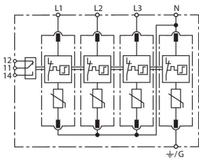
Prinzipschaltbild DG MU 3PY 480 4W+G R
