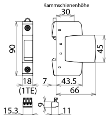
Maßbild DG S 275 VA FM
