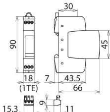
Maßbild DR M 2P 75 FM
