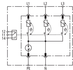
Prinzipschaltbild DR M 4P 255 SN1872 FM
