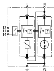
Prinzipschaltbild DG M TT 2P 320 FM
