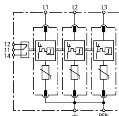
Prinzipialschaltbild DG M TNC 150 FM
