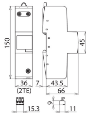
Maßbild DBM 1 760 FM
