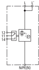
Prinzipialschaltbild DBM 1 760 FM
