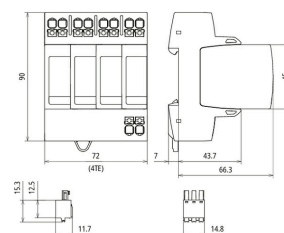
Maßbild DG MP TNS 150 FM
