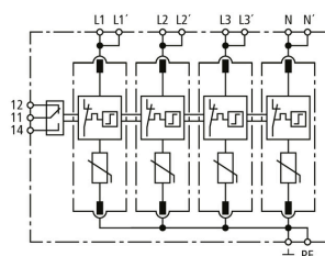
Prinzipialschaltbild DG MP TNS 150 FM
