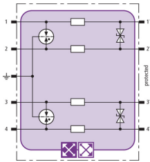
Prinzipialschaltbild BXT ML4 BD 60
