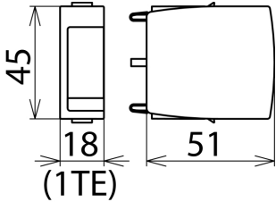
Maßbild DG MOD 150
