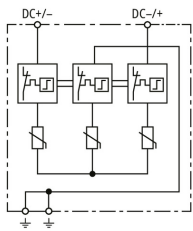
Prinzipschaltbild DCU 2 YPV 1+2 1200 2M 2S MC4
