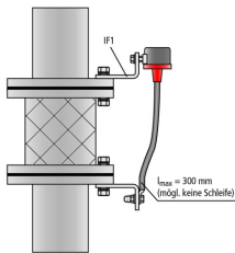
Einbauvariante EXFS L200
