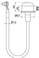
Maßbild EXFS L200
