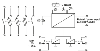
Anschlussschema
